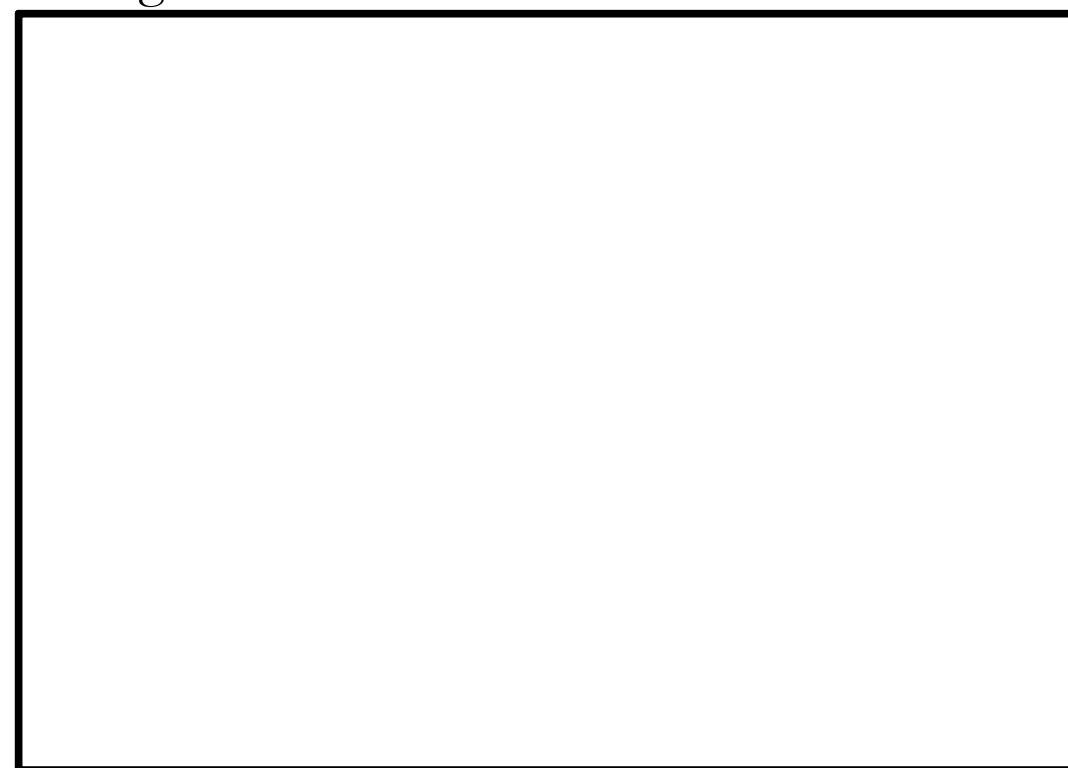
Retângulo de raiz de 2
