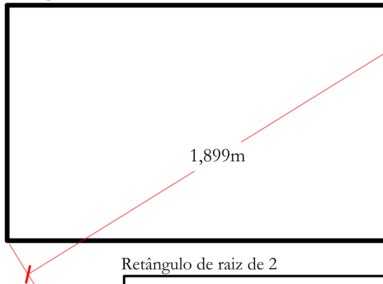
Retângulo de Ouro
